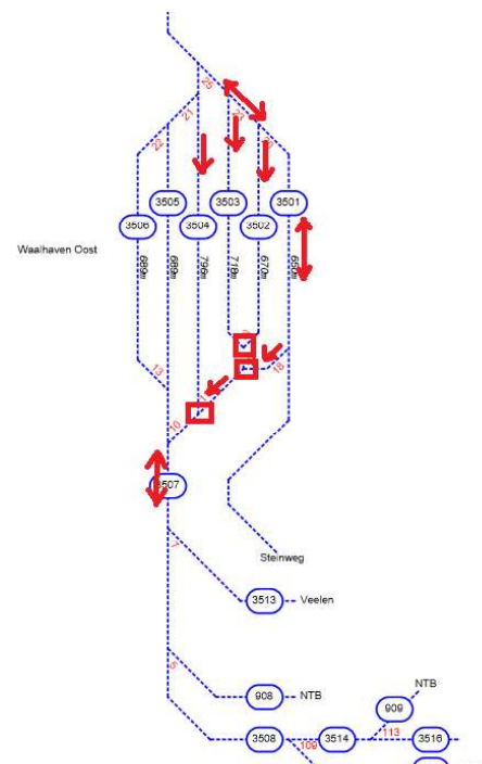
Figuur C.7 Opstelsterrein Waalhaven-Oost
