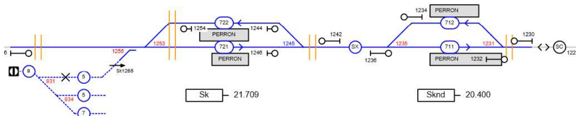
Figuur D.2 Sporenplan van Sneek en Sneek Noord (Sporenplannen, 2021)
