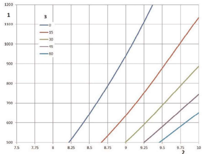
Figuur 3.3 Minimale wieldiameter tegenover invalshoek bij rechte stompe kruising
