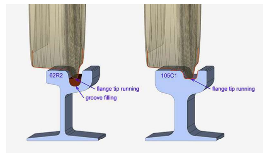
Figuur 2.12 Doorsnede groefrails (Constantin, 2016)
