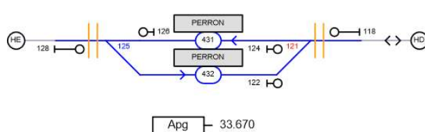
Figuur D.6 Sporenplan van Appingedam (Sporenplannen, 2021)
