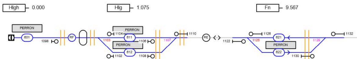
Figuur D.3 Sporenplan Harlingen en Franeke (Sporenplannen, 2021)
