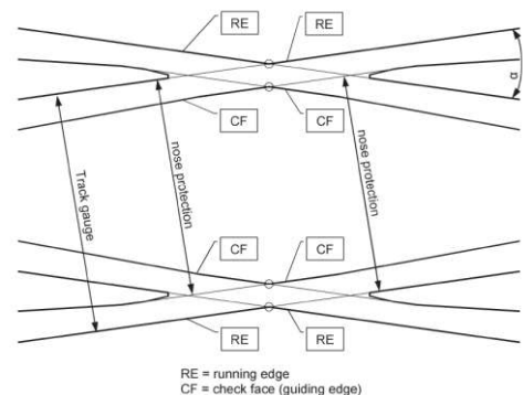
Figuur 3.1 Stompe kruising; met aangegeven strijkregels en bereden spoor
