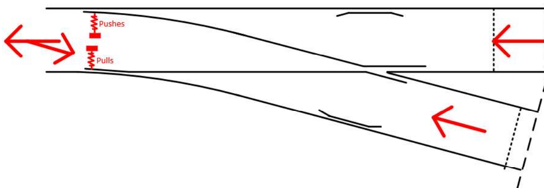
Figuur B.3 Terugklapwissel-principe
