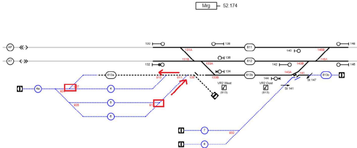
Figuur C.8 Opstelsterrein Maarn
