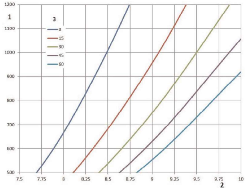
Figuur 3.2 Minimale wieldiameter tegenover invalshoek bij 450 [m] radius stompe kruising
