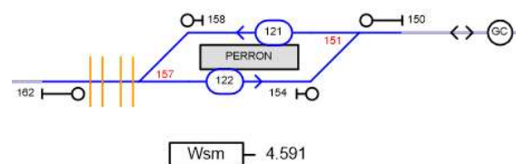
Figuur D.7 Sporenplan van Winsum (Sporenplannen, 2021)
